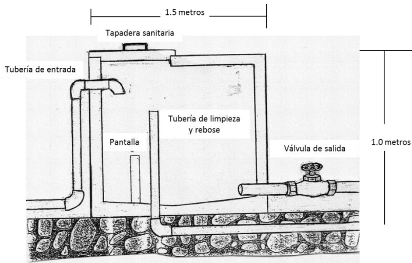
Cámara rompe carga
