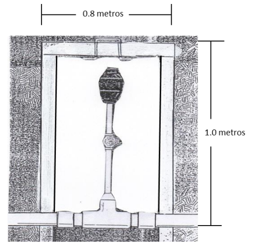
Válvula de aire
